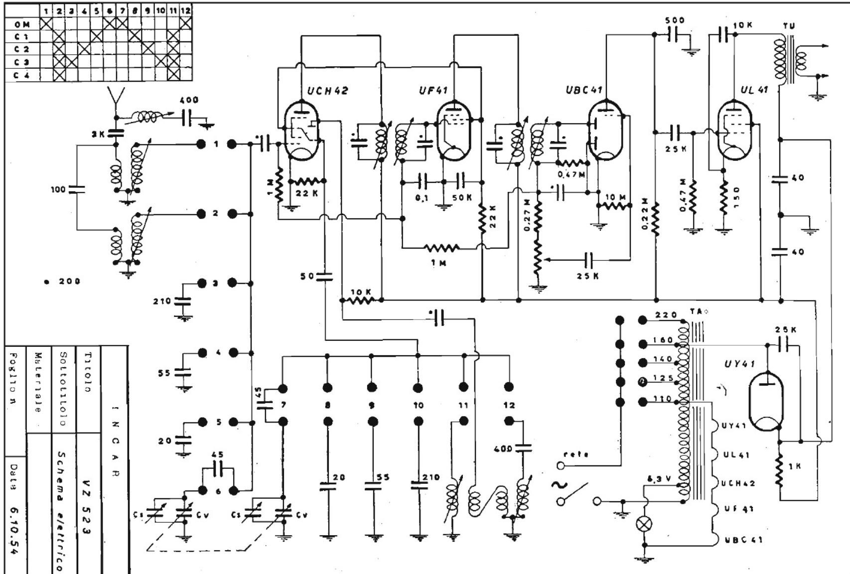
INCAR - Mod. VZ 523. Ricevitore a onde medie con quattro bande allargate ad onde corte. Potenza d'uscita 3 watt. Consumo 50 watt.
